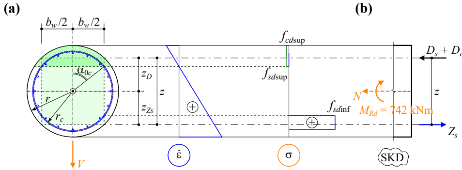
Abbildung 6.4: Theoretische Stegbreite und Hebelarm am reduzierten Querschnitt: (a) Querschnitt; (b) Schnittkörperdiagramm.
