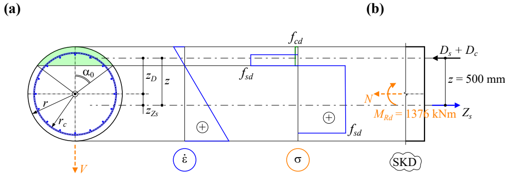
Abbildung 6.3: Biegewiderstand am gesamten Querschnitt: (a) Querschnitt; (b) Schnittkörperdiagramm.
