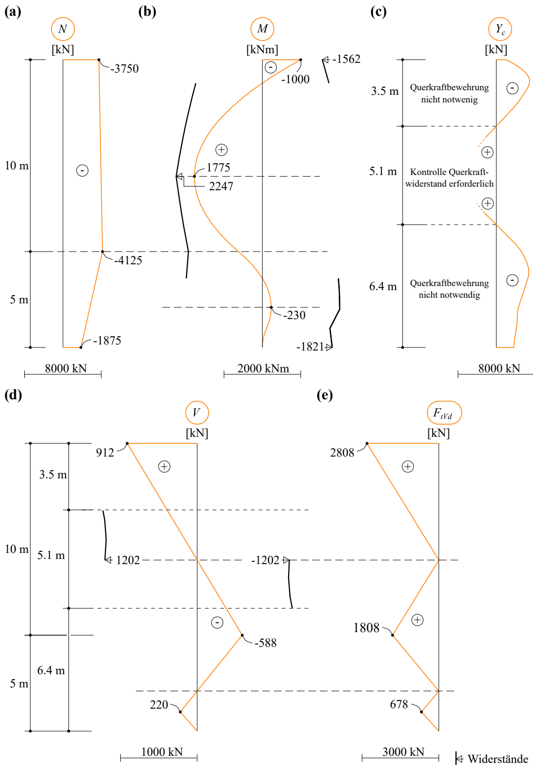
Abbildung 6.6: Zustandslinien der Schnittgrössen des Überprüfungsbeispiels: (a) Normalkraft N ; (b) Biegemoment M ; (c) Fließbedingung Y_c ; (d) Querkraft V ; (e) Längszugkraft infolge Querkraft F_{tVd} .
