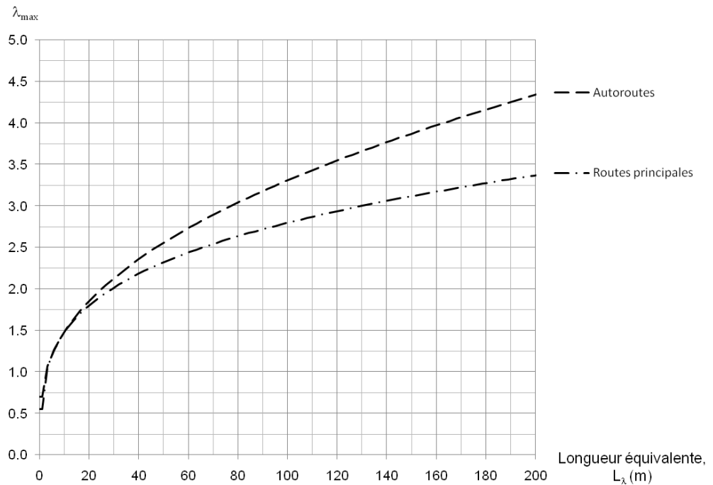
Figure 25: Facteur global d'équivalence de dommage \lambda_{max} pour le trafic routier (extrapolation à partir des résultats de ce travail)
