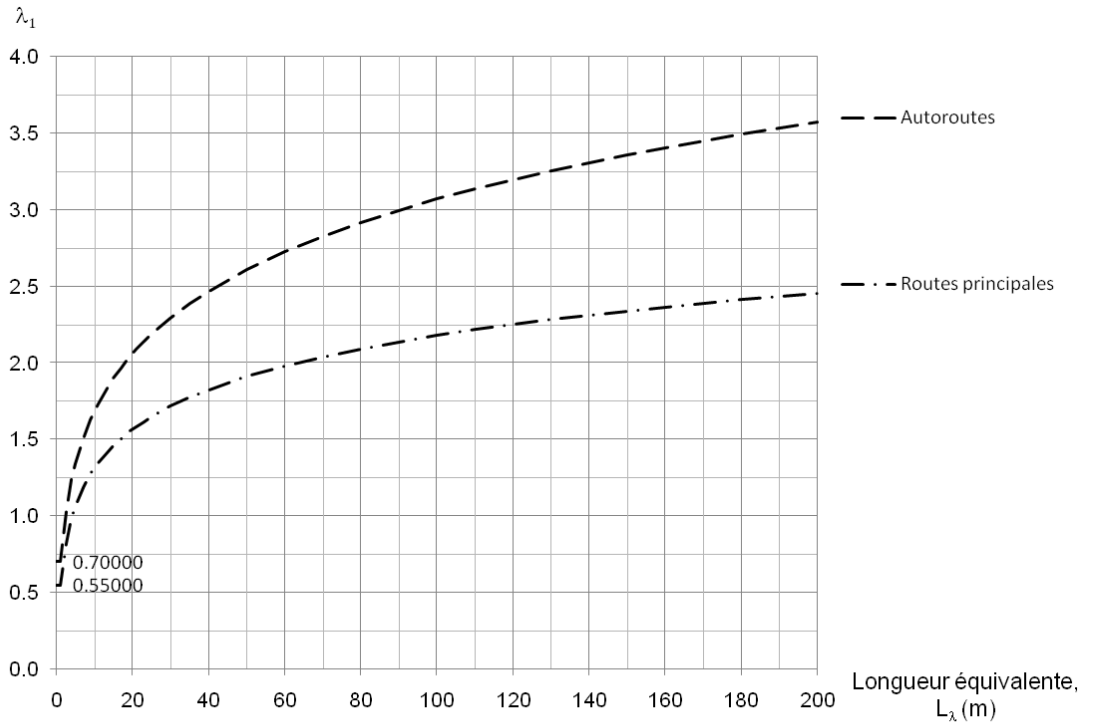
Figure 24: Facteur partiel \lambda_1 pour le trafic routier (extrapolation à partir des résultats de ce travail)
