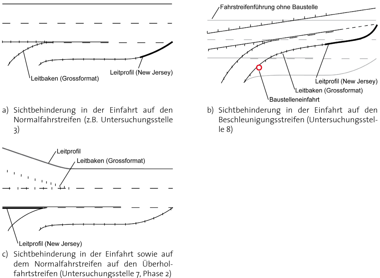
Abbildung 27: Schematische Darstellung der Sichtprobleme bei Einfahrten und Fahrbahnezusammenführungen
