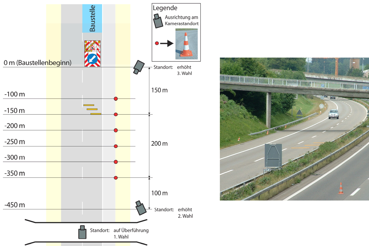
Abbildung 6: Kamerastandorte für Videoaufnahmen und Beispiel eines Aufnahmeortes
