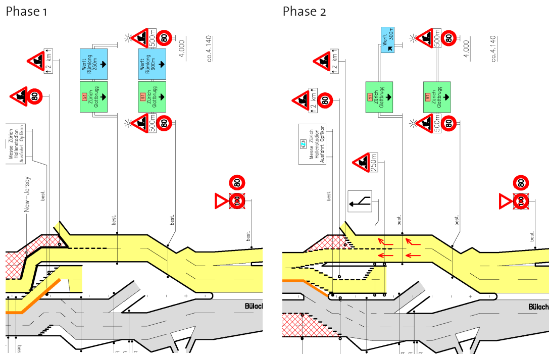
Abbildung 31: Signalisation Untersuchungsstelle 9, Phase 1 und Phase 2
