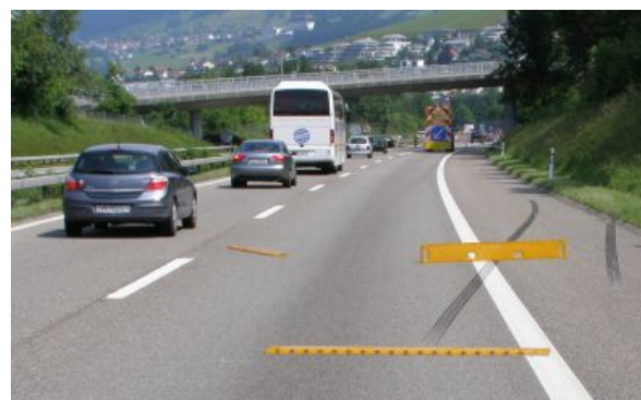
Abbildung 17: Beispiele von grossen Verschiebungen der Warnschwellen
