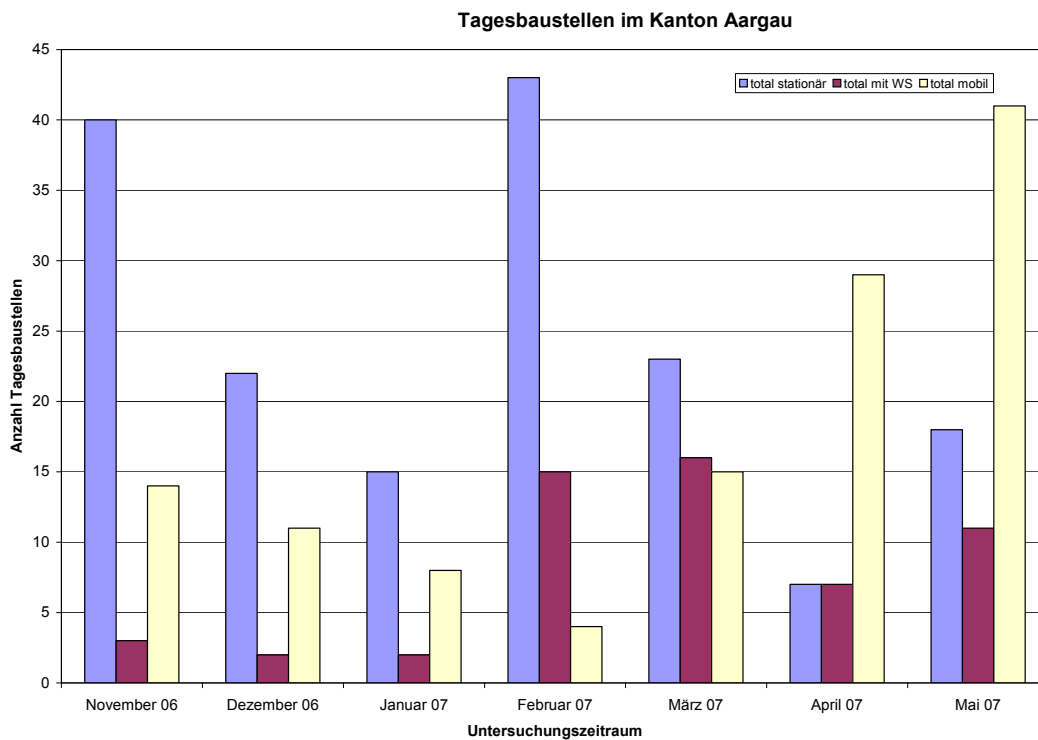
Abbildung 12: Zeitliche Verteilung der Tagesbaustellen und der Warnschwelleinsätze im Kanton Aargau
