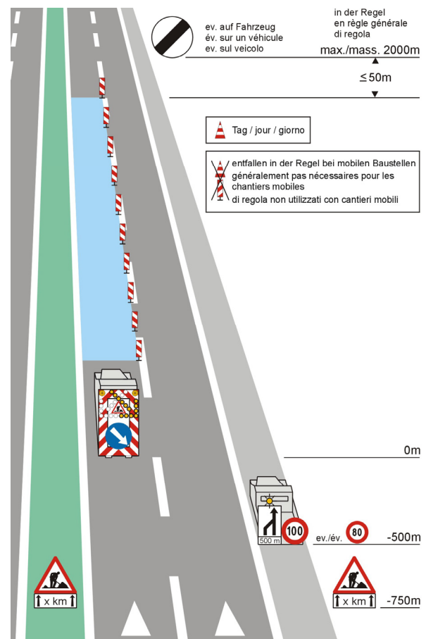
Abbildung 10: SN-Normfigur 12 nach SN 640 885c - Beilage
