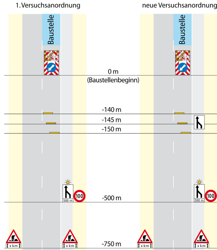
Abbildung 3: Prinzipische Skizze der gewählten Versuchsanordnung
