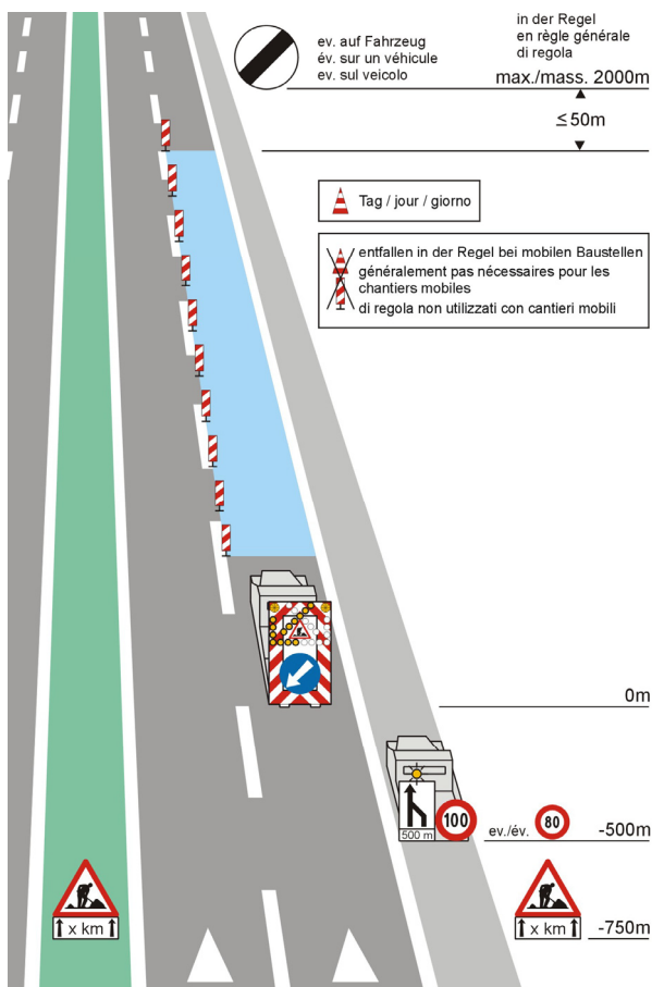
Abbildung 9: SN-Normfigur 10 nach SN 640 885c - Beilage
