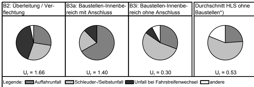
Abbildung 22: Unfalltypen und Unfallraten in ausgewählten Baustellenabschnitten, A1 Limmattal (ZH) und an HLS ohne Baustellen [SPACEK et al. (2005)]
