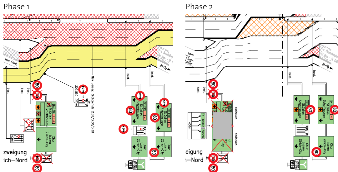
Abbildung 30: Signalisation Untersuchungsstelle 2, Phase 1 und Phase 2
