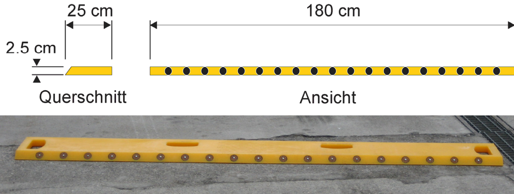
Abbildung 5: Abmessungen und Fotoansicht der eingesetzten Warnschwellen
