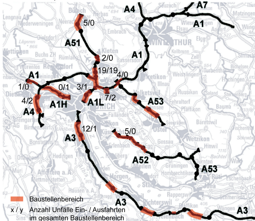
Abbildung 24: Verteilung der Unfälle bei Ein- und Ausfahrten auf die Baustellenbereiche
