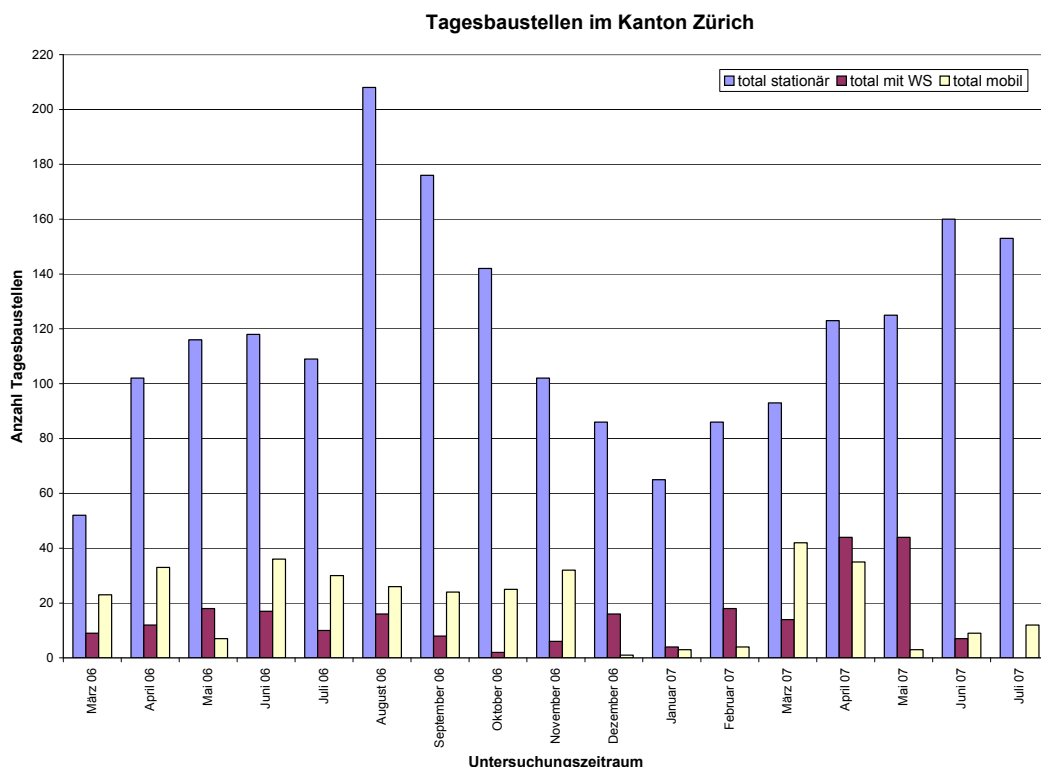
Abbildung 11: Zeitliche Verteilung der Tagesbaustellen und der Warnschwelleinsätze auf den Autobahnen im Kanton Zürich
