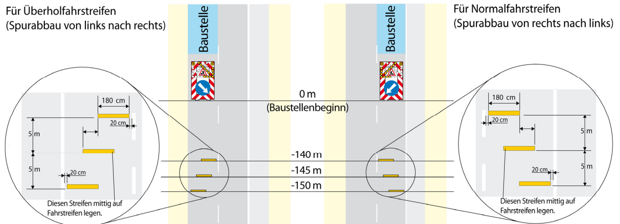
Abbildung 4: Anordnung der Warnschwellen auf dem Fahrstreifen
