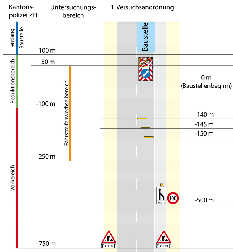
Abbildung 7: Untersucher Bereich des Fahrstreifenwechsels
