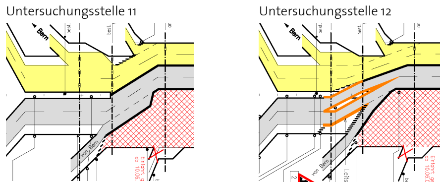
Abbildung 29: Baustellenbetriebsformen der Untersuchungsstellen 11 und 12
