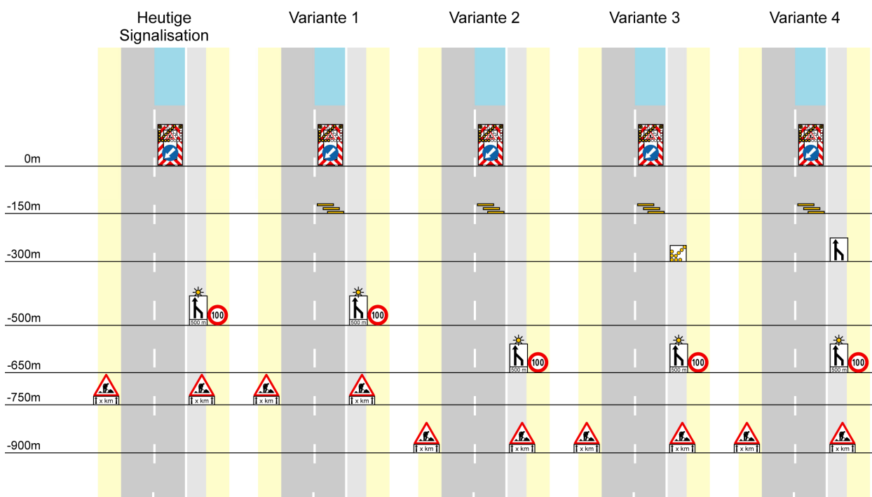
Abbildung 2: Varianten mit schematischer Darstellung der Versuchsanordnung
