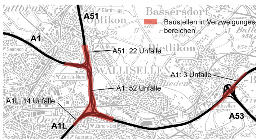
Abbildung 25: Verteilung der Unfälle bei Verzweigungen
