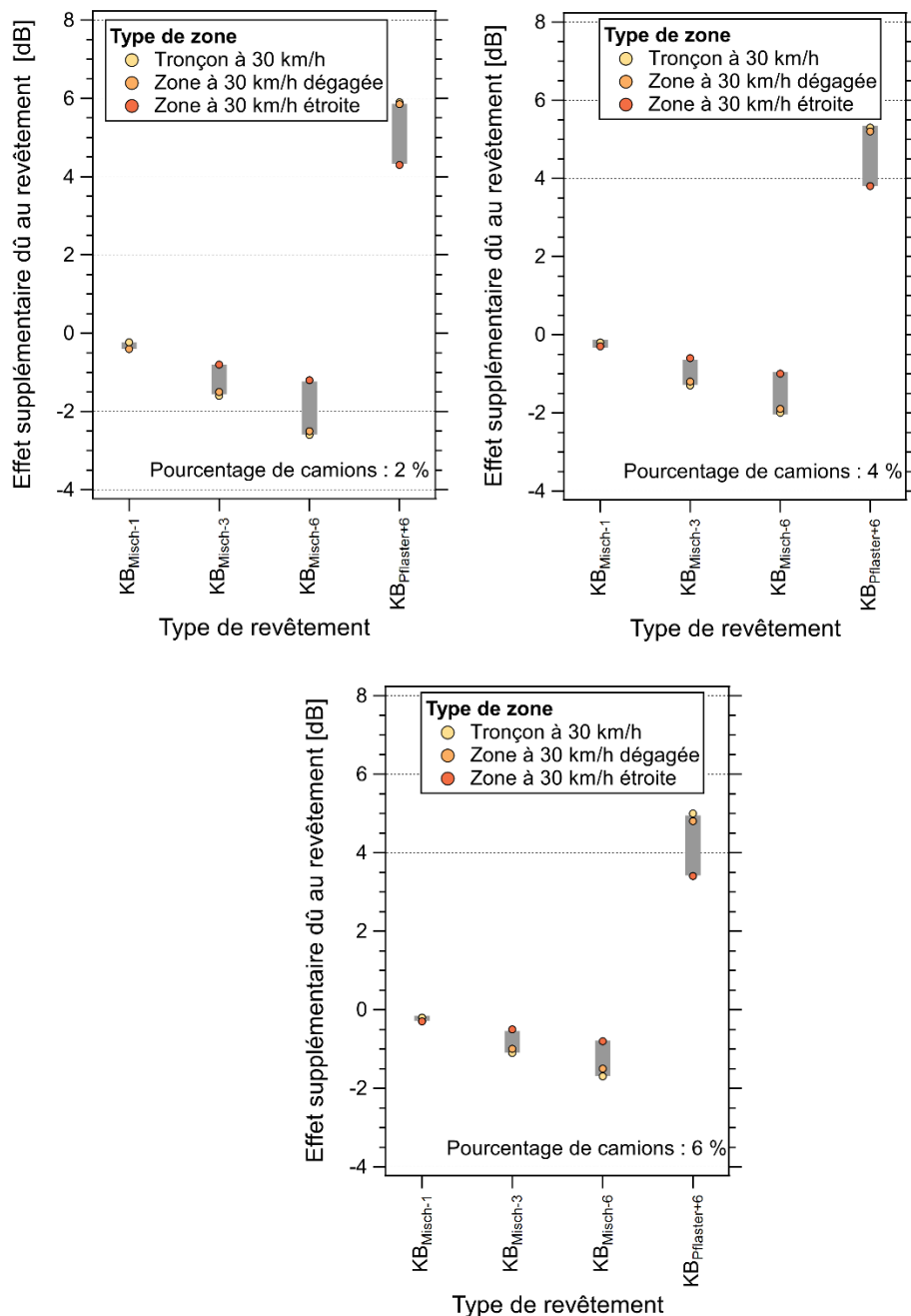
Figure 21 : Impact acoustique supplémentaire prévisible pour plusieurs revêtements cibles possédant différentes valeurs caractéristiques (kb), avec une proportion de camions de 2, 4 et 6 %. La situation initiale est celle d'une limitation de vitesse à 30 km/h avec vitesse moyenne selon le type de zone et un revêtement acoustiquement neutre.
