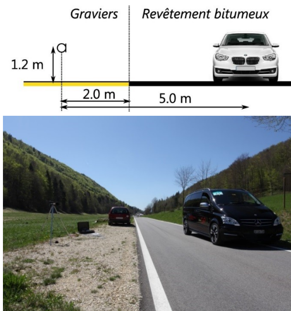
Figure 8 : Dispositif pour mesurages à l'arrêt.
