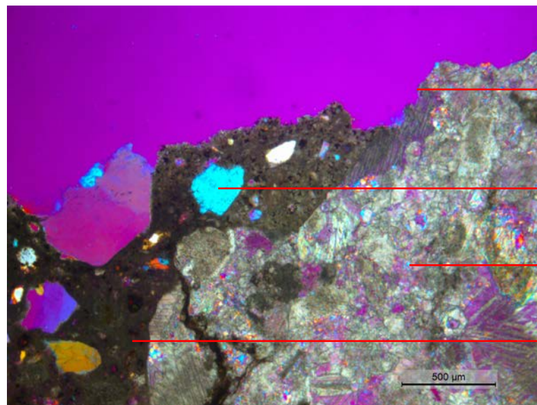
Abb. 27 Mikroskopische Gefügeaufnahme im Polarisationslicht. Beton 7 und 8.
