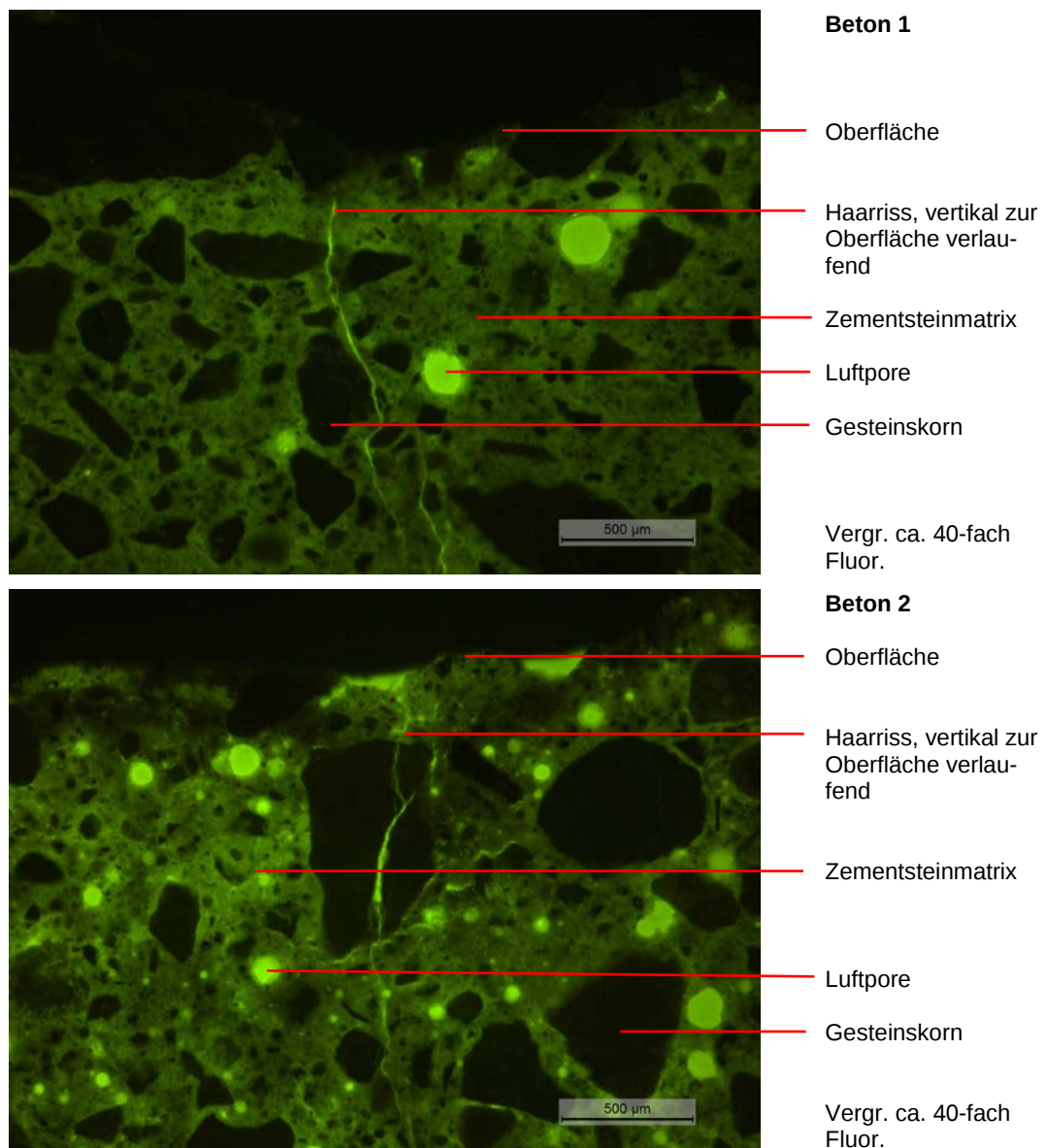
Abb. 24 Mikroskopische Gefügaufnahme im Fluoreszenzlicht. Beton 1 und 2.
