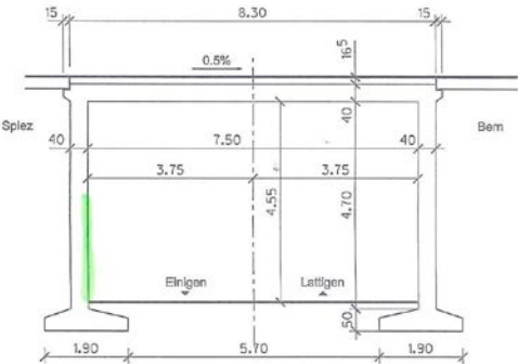
Querschnitt 1:100
