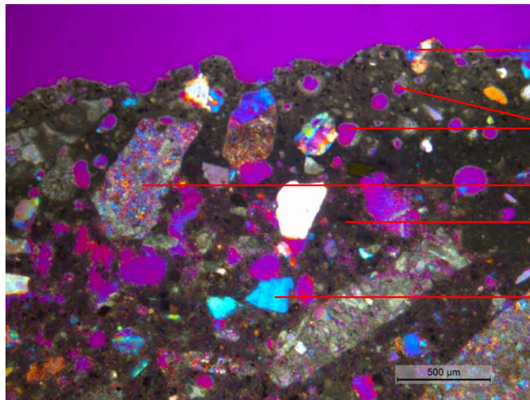
Abb. 25 Mikroskopische Gefügeaufnahme im Polarisationslicht. Beton 3 und 4.
