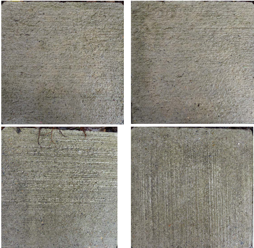
Abb. 19 Zustand der Versuchsplatten am 14.05.2014. Oben: Beton 3. Unten: Beton 8 (jeweils linke und rechte Platte, Blickrichtung Südwesten).
