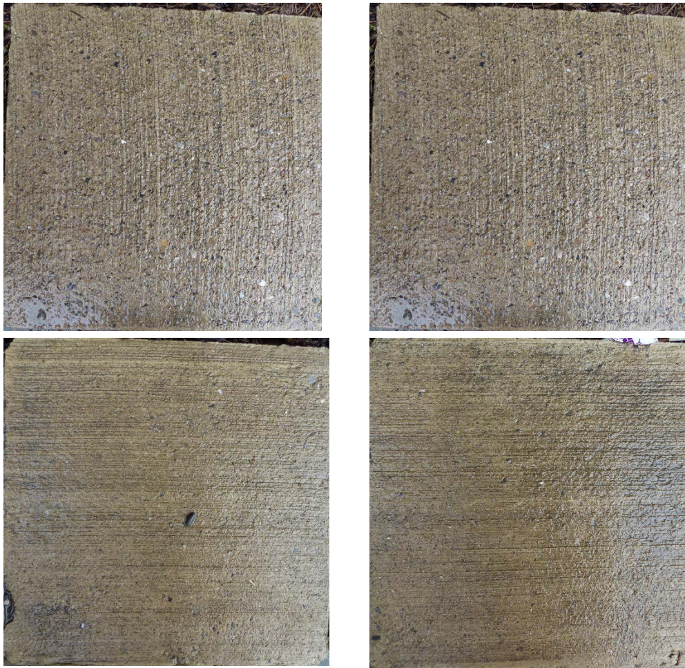
Abb. 21 Zustand der Versuchsplatten der Betone mit CEM III/B und einem w/z-Wert von 0.45 am 14.05.2014. Oben: Beton 9 ohne LP. Unten: Beton 10 mit LP (jeweils linke und rechte Platte, Blickrichtung Südwesten).
