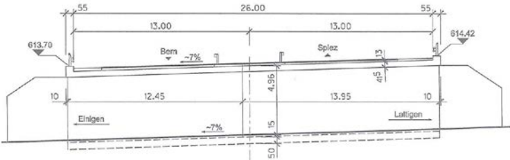
Längsschnitt 1:200
