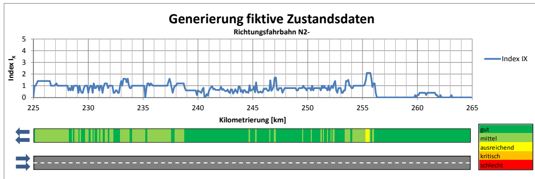
Abb. 31 Fiktive Zustandsdaten Index I_x für das Fallbeispiel der Richtungsfahrbahn N2-
