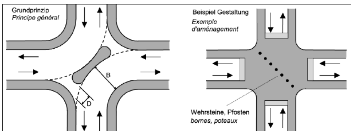
Abb. 3.6: Sperre (Quelle: SN 640 213)
