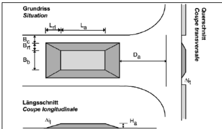
Abb. 3.2: Viereckförmiger Vertikalversatz, „Kissen“ (Quelle: SN 640 213)
