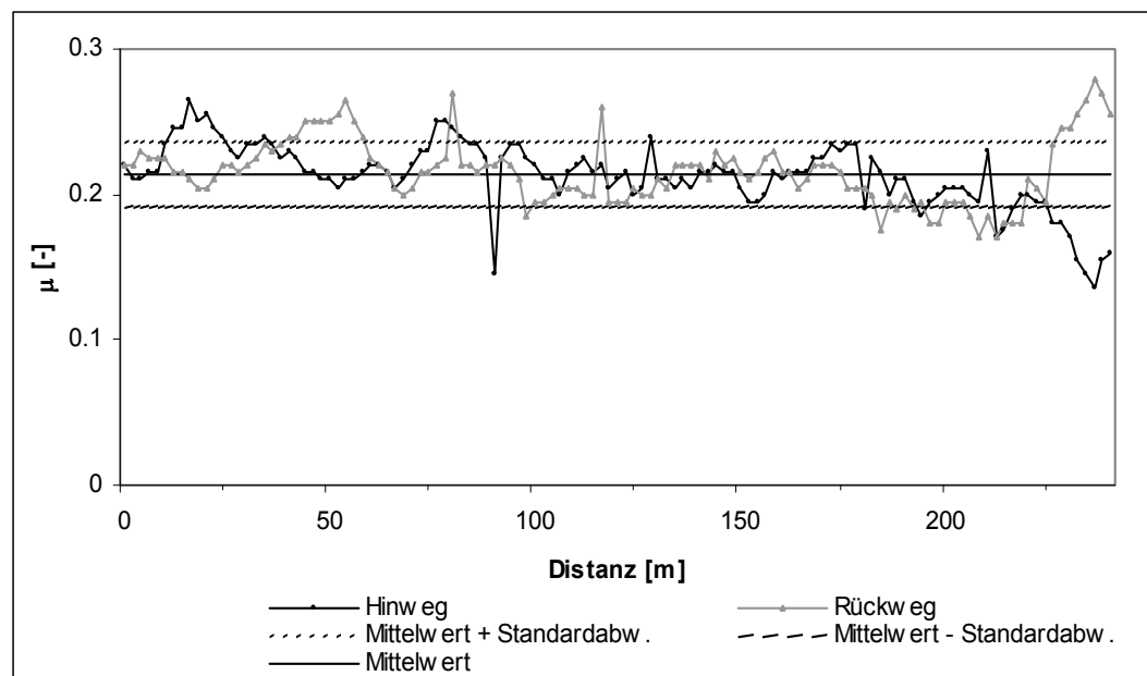
Abb. 5.5 Auswertung Skiddometermessfahrt 7
