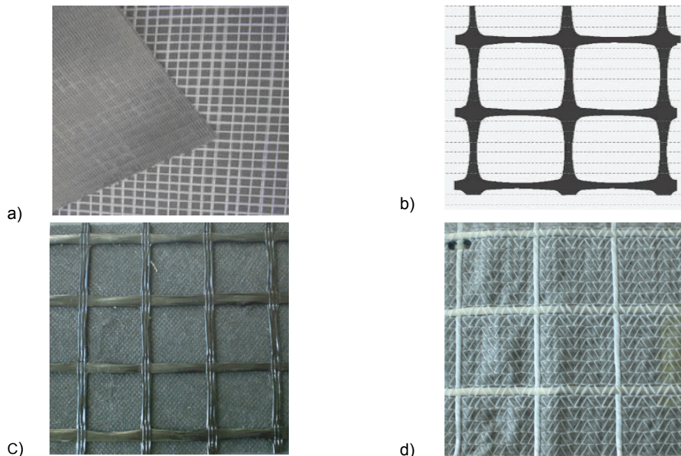
Abb. 2.11 a) Glasfaser auf Vlies geklebt, b) Kunststoffgitter auf Vlies geklebt c) vorbituiniertes Glasfasergitter auf Vlies geklebt d) Glasfaser auf Vlies gewebt; (Asphalt Academy, 2008)
