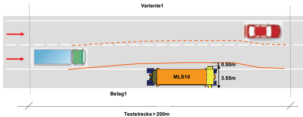
Abb. 6.43 Teststrecke mit vorhandenen oder künstlich erzeugten Schäden bei ausreichenden Platzverhältnissen (schematisch, nicht massstäblich) Festlungen nach VSS-Normen (SN 640 885c, 1999) und ASTRA-Richtlinie (Art. Nr. 308 103.d, 2002))
