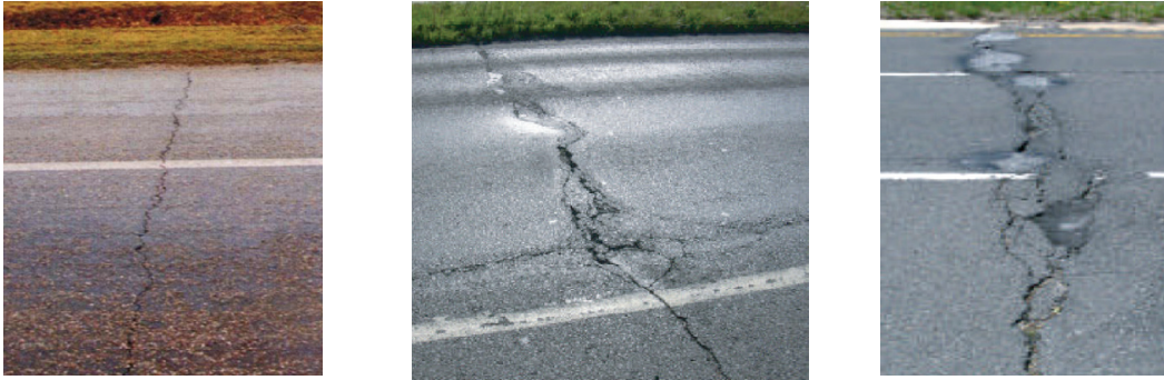
Abb. 2.3 Typische Schadensbilder für Reflexionsrisse (Bennert und Maher, 2008; Rathmeyer, 2007)
